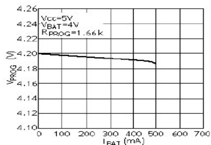
稳定输出（浮充）电压与充电电流的关系曲线
